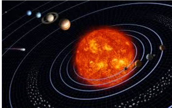
sistema solare “centro mosso”
