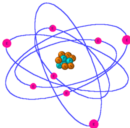
representazione dell' atomo: le orbite degli elettroni E, sono vortici!
